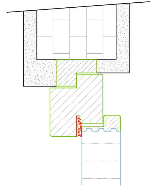
Stockrahmentür mit Überschlag
